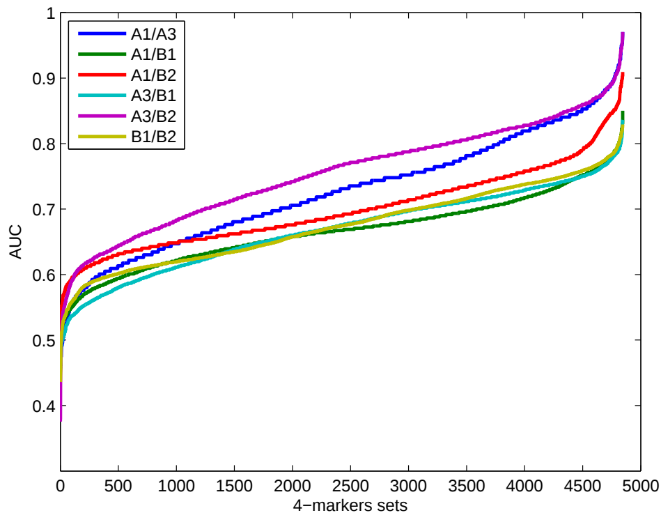
Рис. 1. Для всевозможных наборов из четырех маркеров вычислено значение AUC (для каждой пары классов). На графике отложены эти значения в порядке возрастания. Обратим внимание на то, что значение по оси абсцисс — не более чем порядковый номер значения AUC, не привязанный ни к какому определенному набору маркеров.
