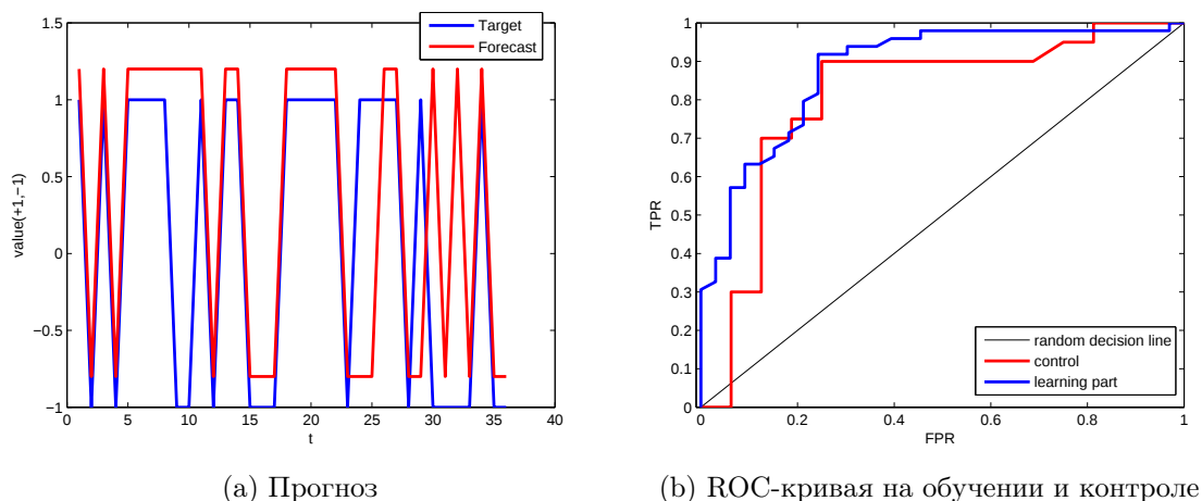
Рис. 6. Результаты при b = 11 : Error = 19\% , AUC_1 = 0,88 , AUC_2 = 0,80
