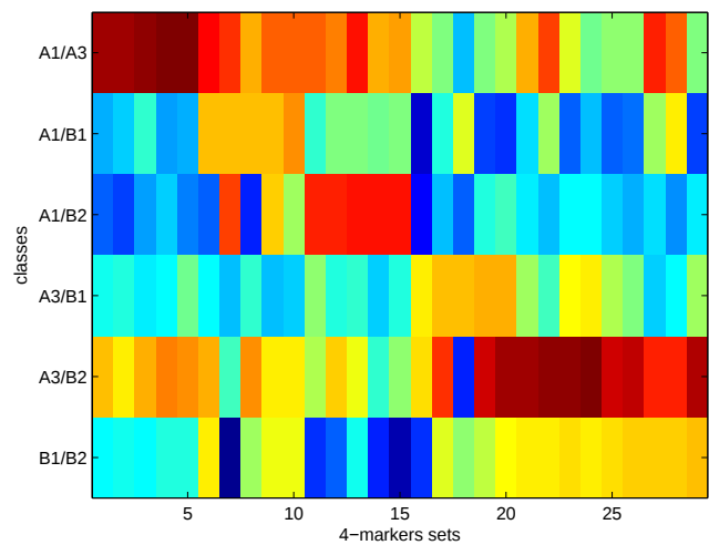
Рис. 3. Для каждого из 30 полученных наборов наиболее информативных признаков приведено его значение AUC (для каждой пары классов).
