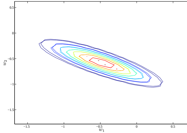
Рис. 5. Контурный график ее аппроксимации Лапласа с ковариационной матрицей общего вида.
