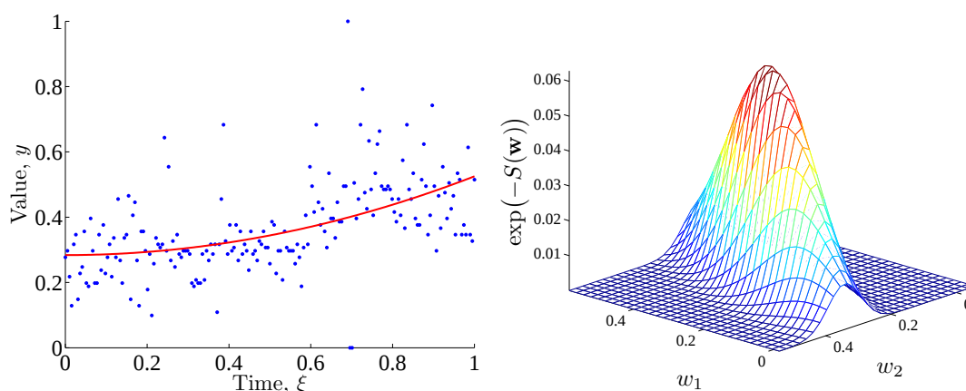
Рис. 1. Аппроксимация данных с помощью функции f(x, w) = w_1 + w_2 * x^2 при оптимальных значениях параметров w = w_{MP} и ненормированная функции ошибки \exp(-S(w)) в окрестности w = w_{MP} .
