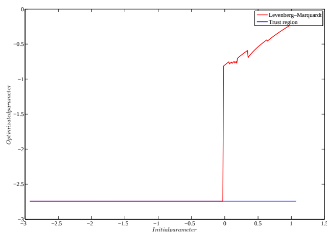
Рис. 6. Зависимость значения параметра h_0 , полученного в результате оптимизации от его начального значения.
