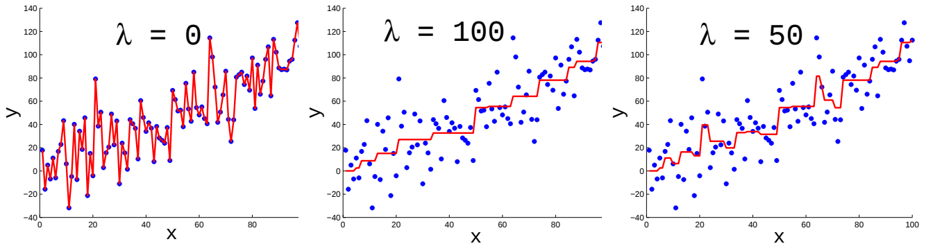
Рис. 1. Монотонная интерполяция
