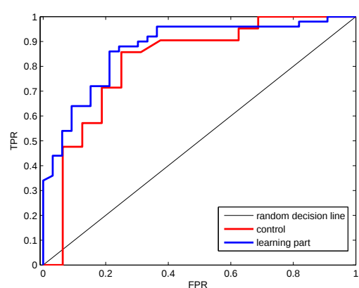
(b) ROC-кривая на обучении и контроле
