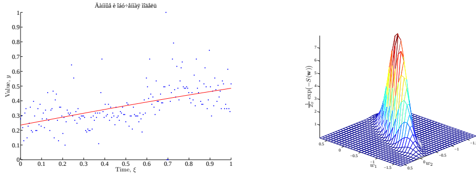
Рис. 4. Аппроксимация данных с помощью функции f(x, w) = \frac{1 - \exp(w_1 + w_2 * x)}{1 + \exp(w_1 + w_2 * x)} при оптимальных значениях параметров w = w_{MP} и ненормированная функции ошибки \exp(-S(w)) в окрестности w = w_{MP} .
