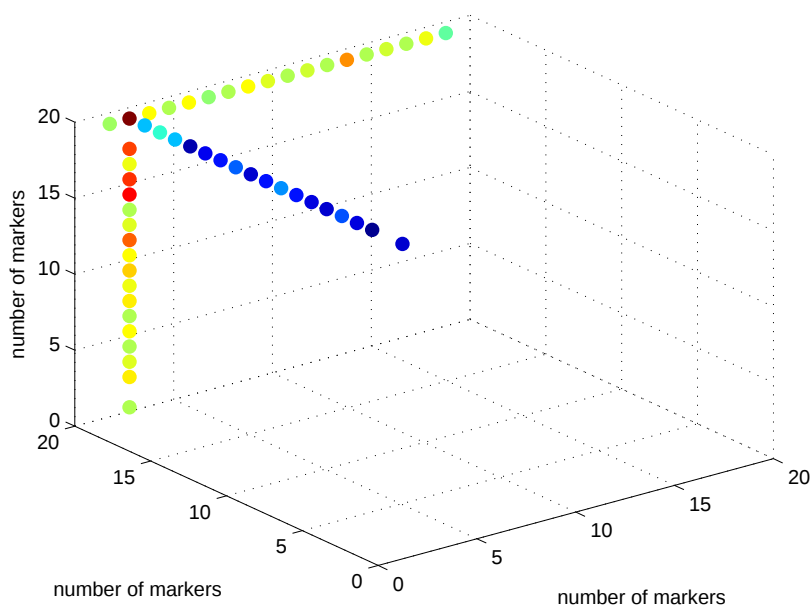
Рис. 4. Оптимальный набор маркеров (2, 19, 20), получаемый при ограничении на сложность модели, равном трем, в окрестности неоптимальных наборов. Чем теплее цвет, тем больше значение оптимизируемого функционала.
