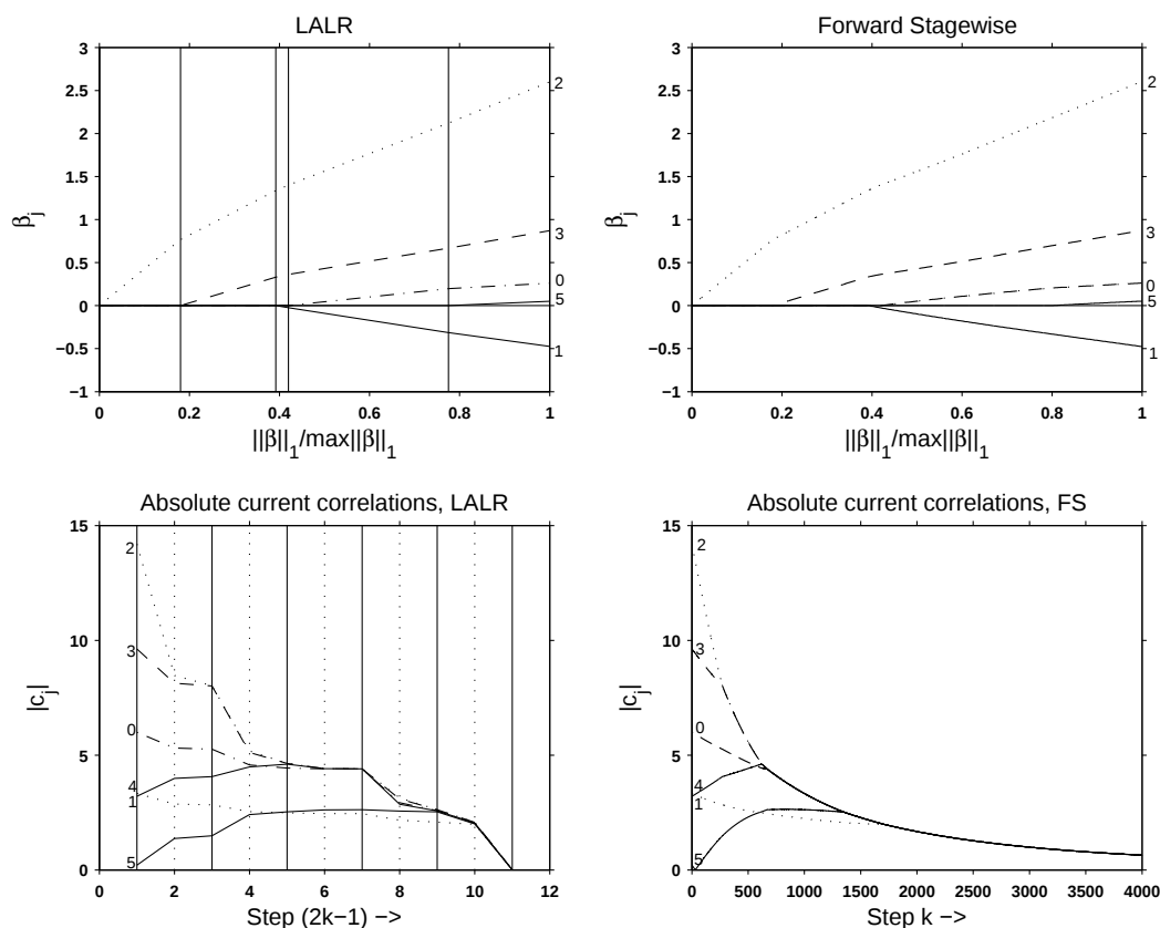
Рис. 2. Сравнение оценок коэффициентов для LALR и Forward Stagewise для модельных данных. Номера кривых соответствуют номерам признаков. Сплошные вертикальные линии обозначают шаги, а штриховые вертикальные — дополнительную итерацию для каждого шага.
