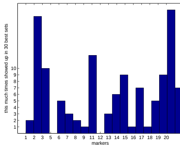
Рис. 2. Количество вхождений каждого из двадцати маркеров в набор « K лучших», \mathcal{S} . Например, маркер под номером 2 (L) имеет наибольшую частоту вхождений, следующий за ним — номер 19 (U/Y).
