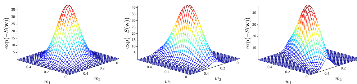
Рис. 2. Аппроксимации с помощью функции нормального распределения с различными видами матрицы ковариаций: с постоянной дисперсией, диагональной и общего вида.
