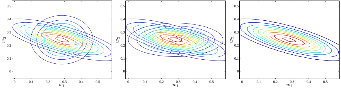
Рис. 3. Сравнение различных типов аппроксимации с реальной функцией ошибки.
