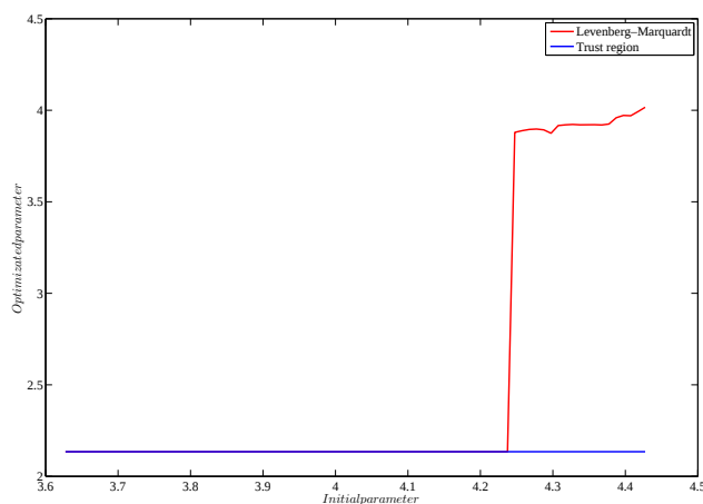
Рис. 7. Зависимость значения параметра h_{22} , полученного в результате оптимизации от его начального значения.
