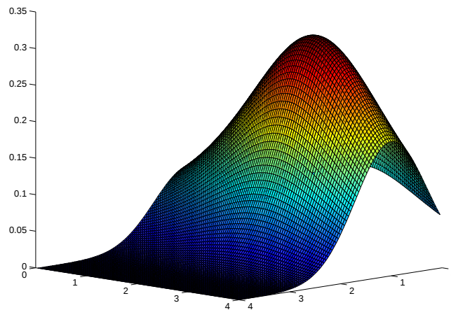
Рис. 10. Функция Котанчека
