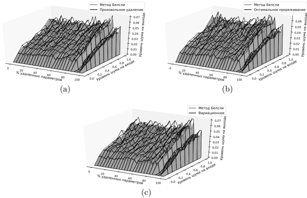
Рис. 3: Влияние шума в начальных данных на шум выхода нейросети на выборке Wine: а) произвольное удаление параметров; б) оптимальное прореживание; с) вариационный метод
