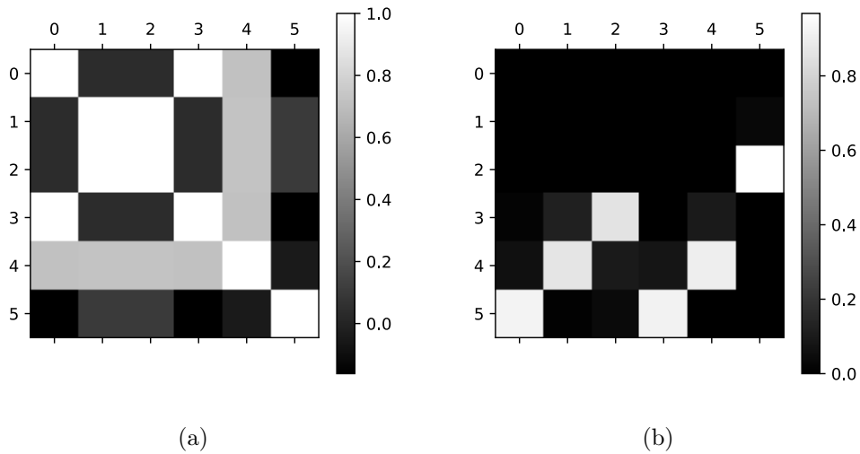
Рис. 1: Иллюстрация метода Белсли: а) матрица ковариации; б) дисперсионные доли
