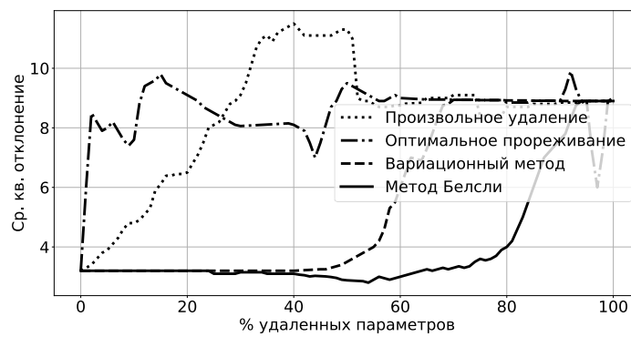
Рис. 4: Качество прогноза при удалении параметров на выборке Boston
