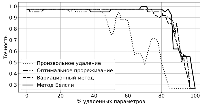
Рис. 2: Качество прогноза при удалении параметров на выборке Wine
