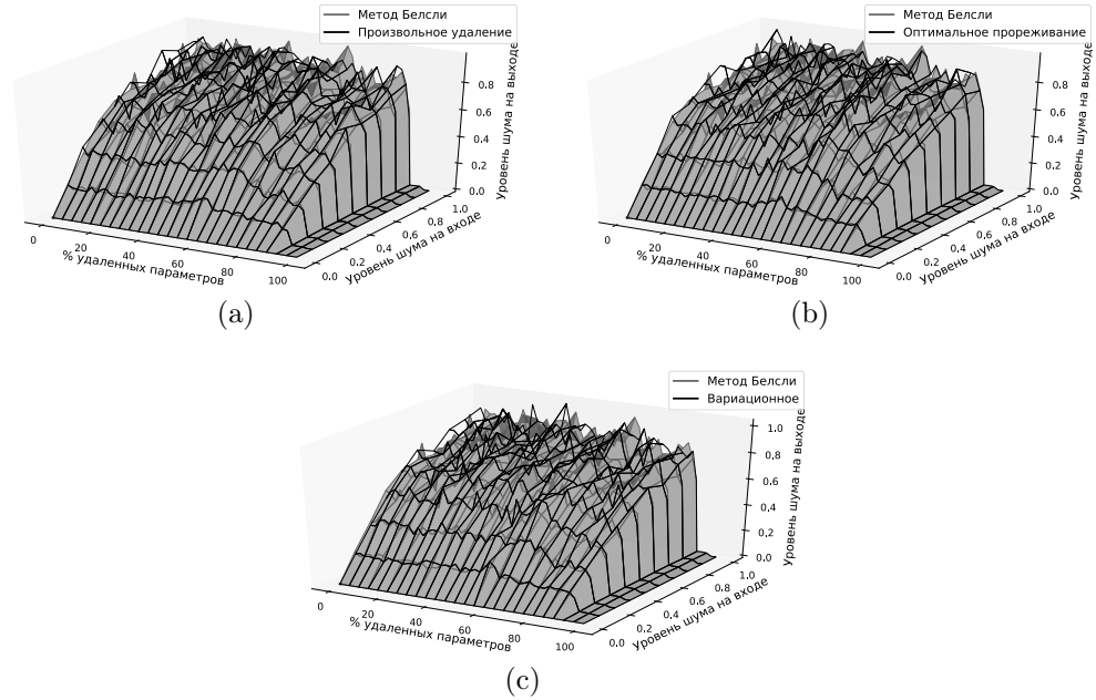
Рис. 5: Влияние шума в начальных данных на шум выхода нейросети на выборке Boston: а) произвольное удаление параметров; б) оптимальное прореживание; в) вариационный метод
