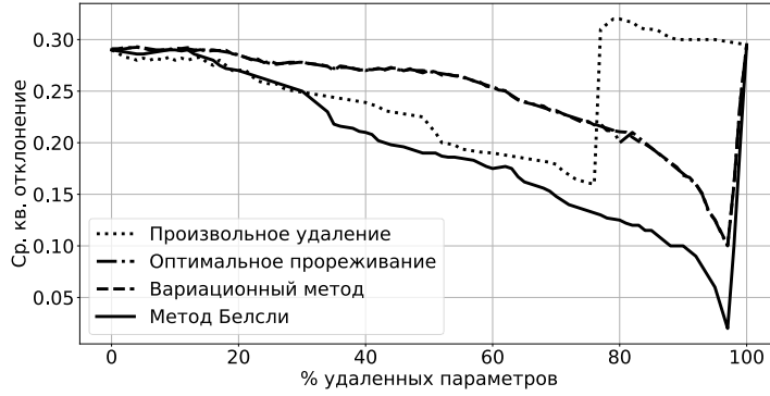
Рис. 6: Качество прогноза при удалении параметров на синтетической выборке
