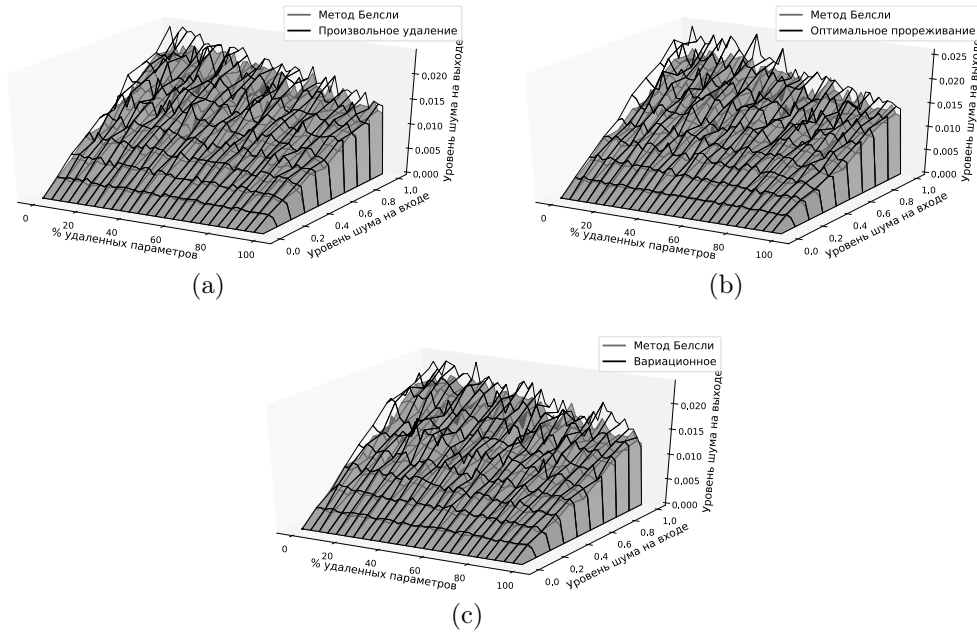
Рис. 7: Влияние шума в начальных данных на шум выхода нейросети на синтетической выборке: а) произвольное удаление параметров; б) оптимальное прореживание; в) вариационный метод
